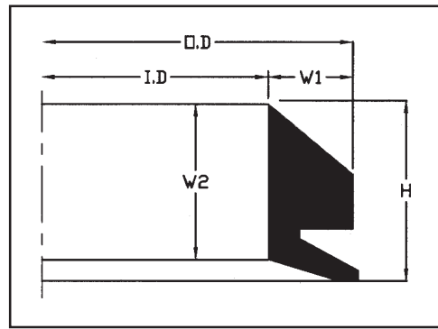
V SEAL : VS TYPE
