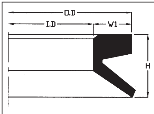
V SEAL : VL TYPE
